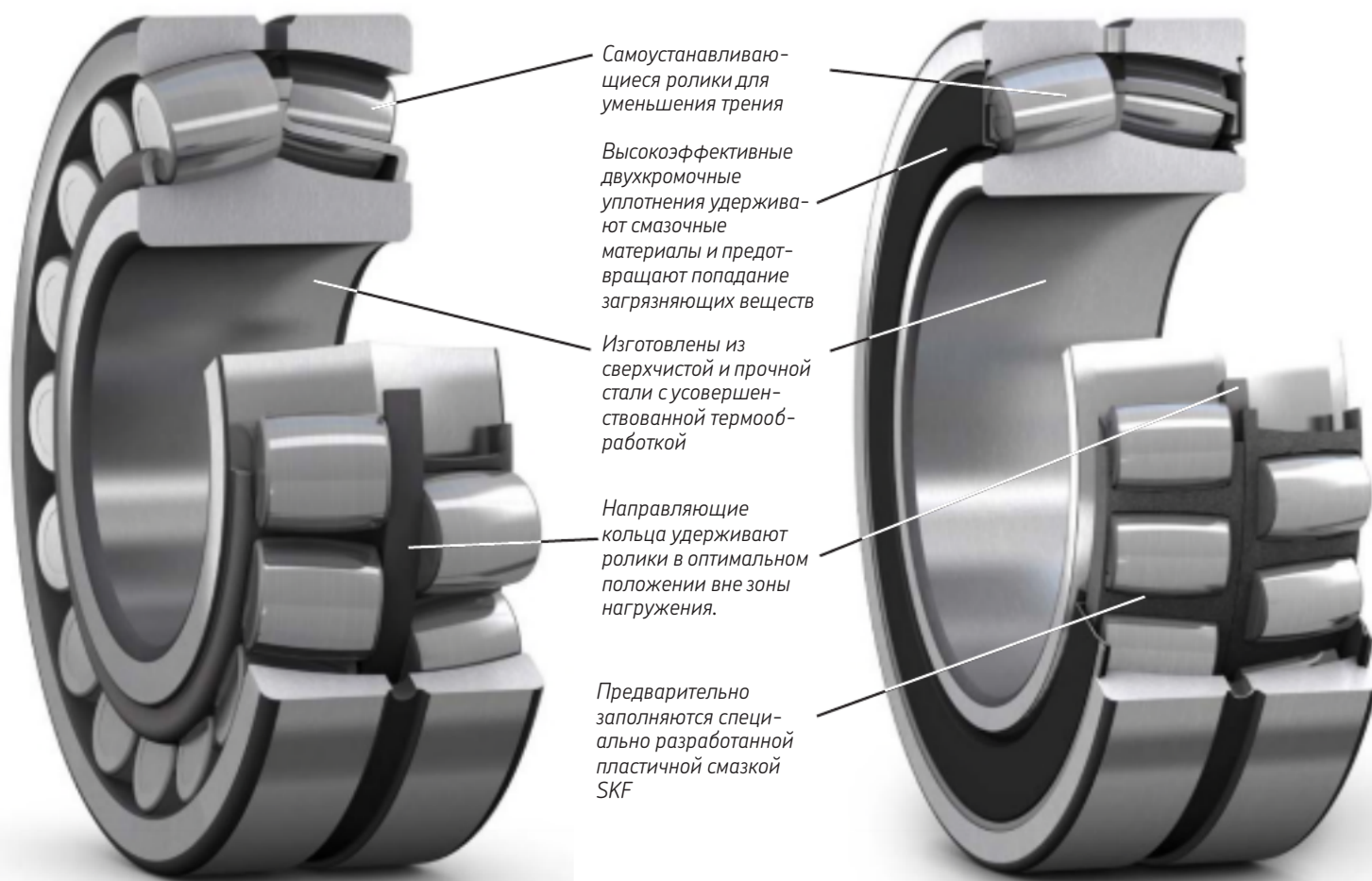
Ресурс подшипника
