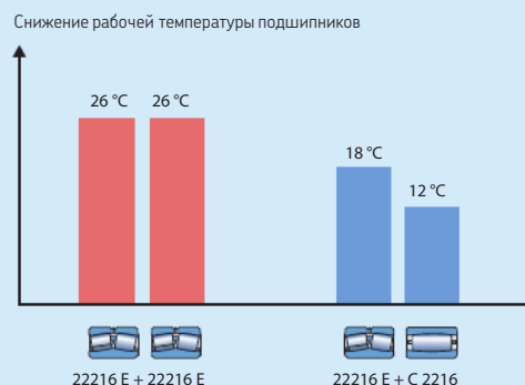
Модернизация промышленного вентилятора — тороидальный роликоподшипник CARB C 2216, смазывание маслом, 3 000 об/мин
