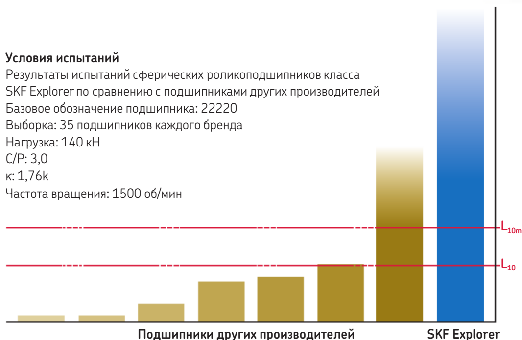
Ресурс подшипника
