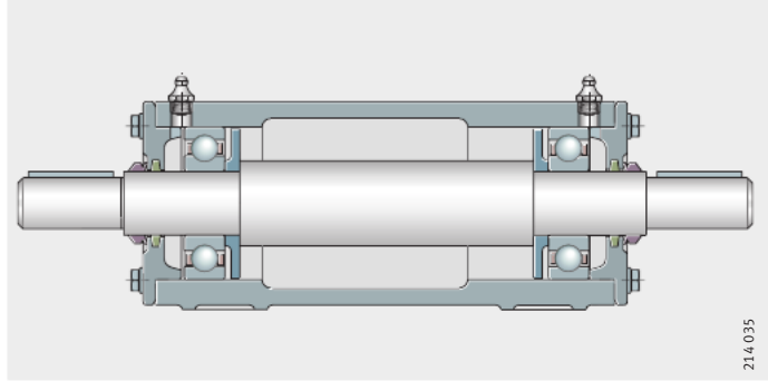
Рисунок 21 Подшипниковый узел VRE3...-A
