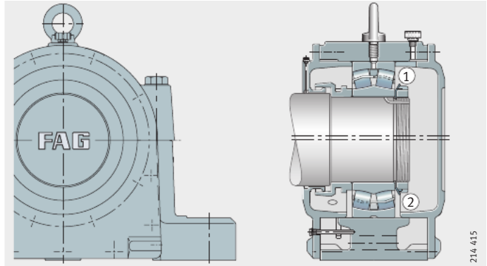
Рисунок 17 Стационарные корпуса LOE2, LOE3, исполнение A
