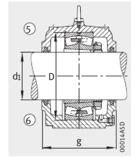
Исполнение В ⑤ фиксир. опора BF ⑥ плавающ. опора BL
