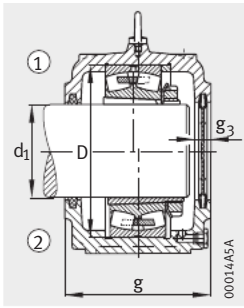
Крышка DK, типоразмеры корпусов до S3040 включ. образуют фиксир. опору при установке упорного кольца
