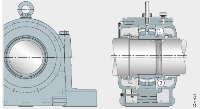
Рисунок 18 Стационарные корпуса LOE2, LOE3, исполнение B
