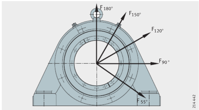
Рисунок 47 Ориентировочные значения разрушающей нагрузки для корпусов BND из стали или модифицированного чугуна
