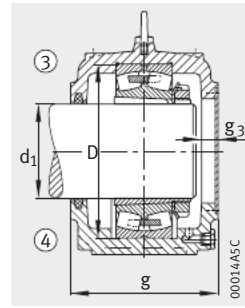
Исполнение А ③ фиксир. опора AF ④ плавающ. опора AL
