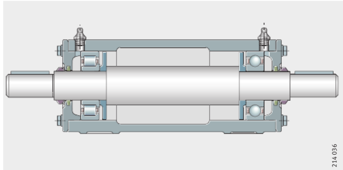
Рисунок 22 Подшипниковый узел VRE3...-B
