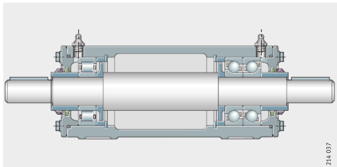
Рисунок 23 Подшипниковый узел VRE3...-C
