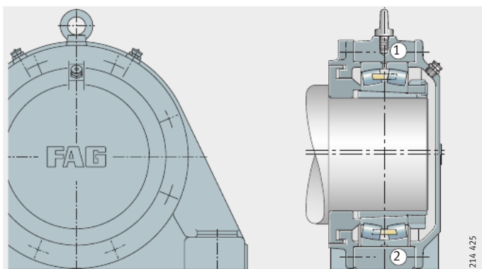
Рисунок 35 Стационарный корпус BND для подшипника с коническим отверстием и закрепительной втулкой и вала с запяточком (лабиринтное уплотнение), исполнение А
